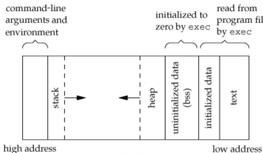
Figure 1: Linux 上的一般執行檔記憶體布局
